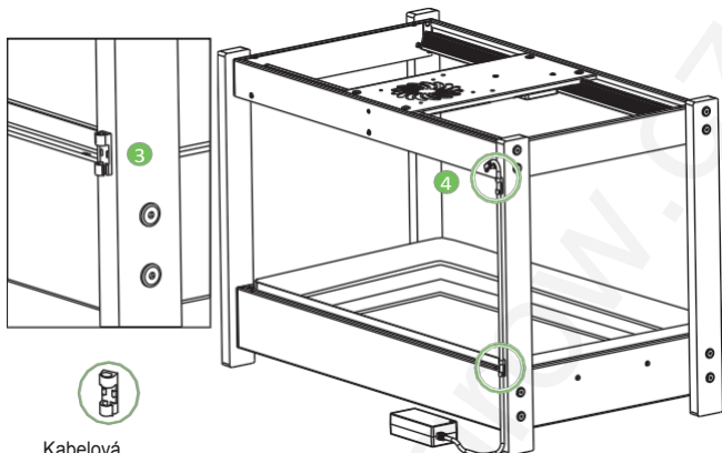
Kabelová svorka 2x
